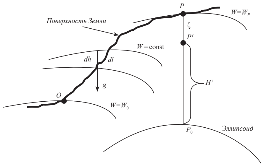
Рис. 4. К определению высоты в поле силы тяжести
