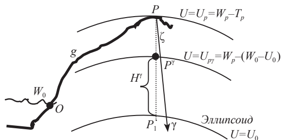
Рис. 3.1. Нормальная высота и аномалия высоты
