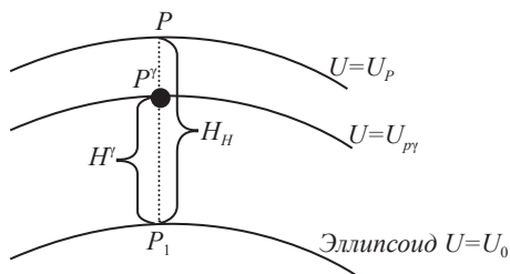
Рис. 3. 2. Высота в нормальном поле и нормальная высота
