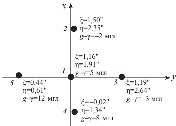
Рис. 4.9. К определению вторых производных (схема расположения вычислительных точек)
