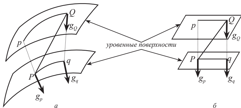
Рис. 1. Уровенные поверхности неоднородного (а) и однородного (б) полей
