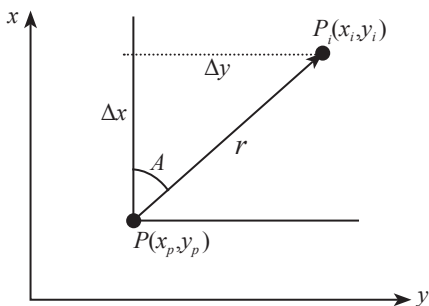
Рис. 3.12. Связь плоских прямоугольных и полярных координат на плоскости z=0 (ось z перпендикулярна к плоскости чертежа)
