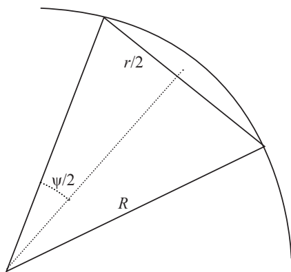
Рис. 3.10. Связь углового и линейного расстояний
