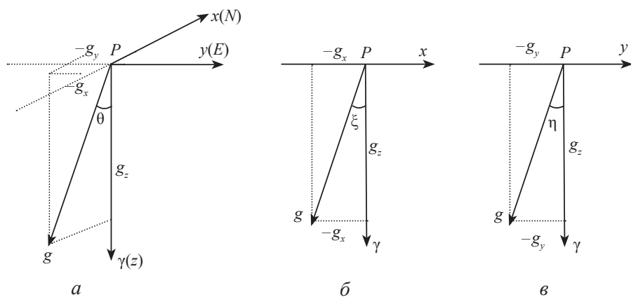
Рис. 2.2. Гравиметрическое уклонение отвеса (а). Составляющая уклонения отвеса в плоскости меридиана (б) и в плоскости первого вертикала (в)
