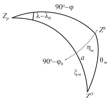
Рис. 4.6. Местное уклонение отвеса
