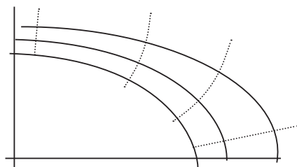
Рис. 1.2. Силовые линии (—) и уровенные поверхности (-----) нормального поля вблизи нормальной Земли
