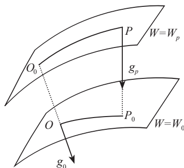
Рис. 4.2. Неоднородное поле
