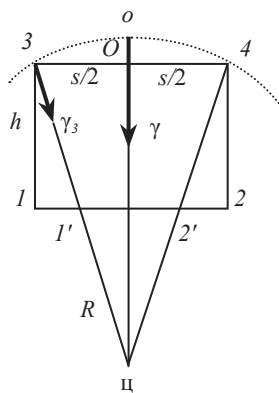
Рис. 4.7. Неоднородность центрального поля
