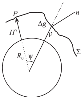
Рис. 3.4. Краевая поверхность в сферическом приближении
