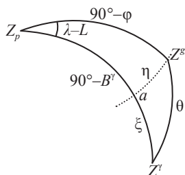
Рис. 2.4. Составляющие гравиметрического уклонения отвеса
