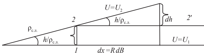
Рис. 1.3. Непараллельность уровенных поверхностей
