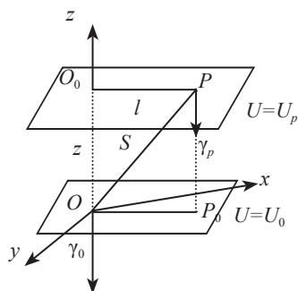
Рис. 4.1. Однородное поле
