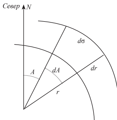
Рис. 3.11. Полярные координаты на плоскости и элемент поверхности
