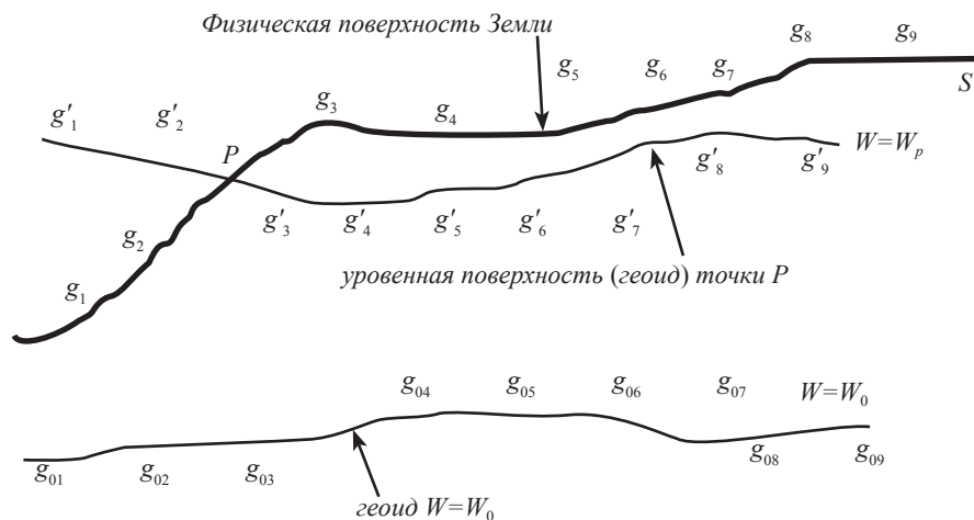
Рис. 3.7. Современная интерпретация задачи и решения Стокса:
