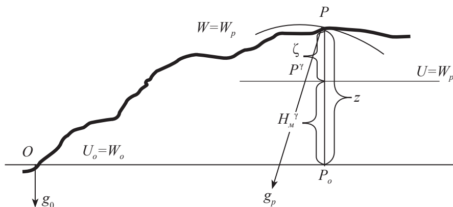
Рис. 4.5. Однородное нормальное поле
