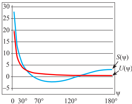
Рис. 3.6. Функции Стокса и Неймана
