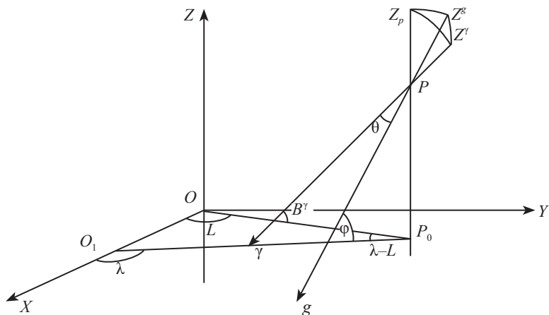
Рис.2.3. К связи натуральной и нормальной систем координат
