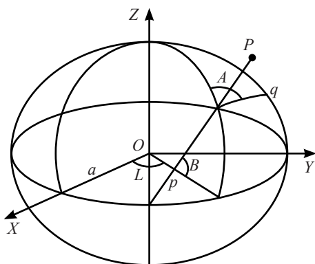
Рис. 2. Геодезические координаты
