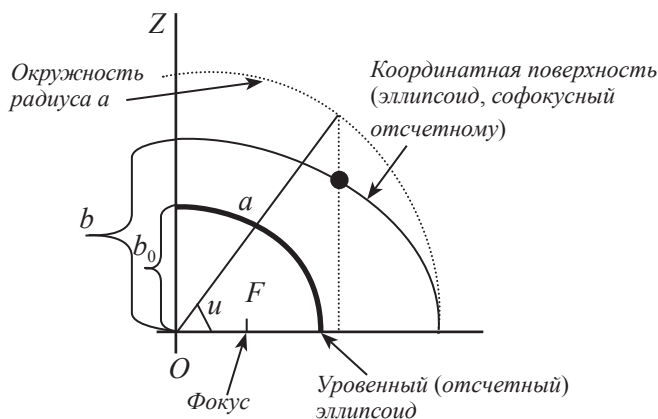
Рис. 1.1. Система координат сжатого эллипсоида
