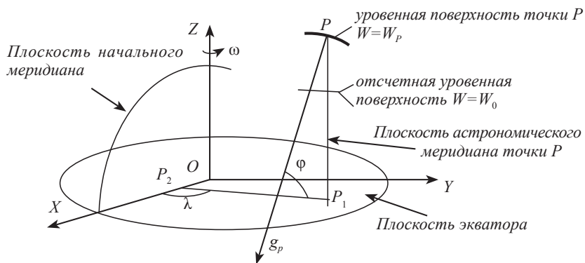
Рис. 3. Астрономические координаты
