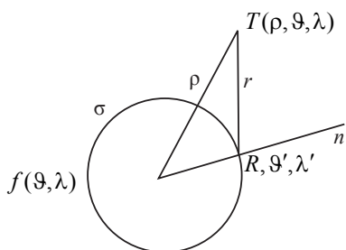
Рис. П1. Сферическая краевая поверхность
