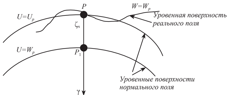
Рис. 2.1. Чистая аномалия высоты
