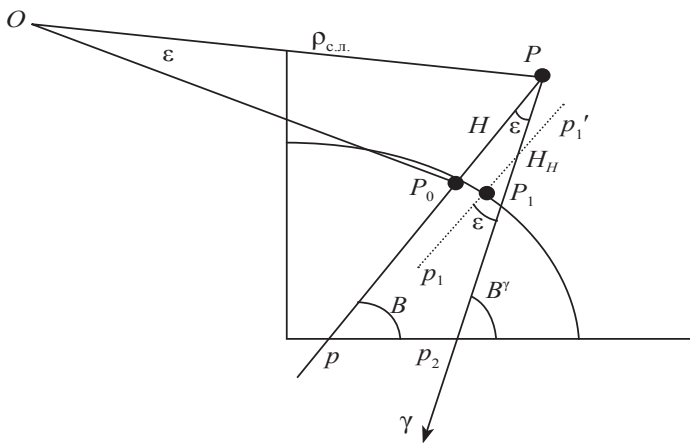
Рис. 1.4. Кривизна силовой линии и система координат в нормальном поле
