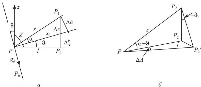
Рис. 4.3. К связи линейных и угловых величин в однородном ( а ) и неоднородном ( б ) поле
