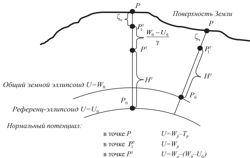
Рис. 3.9. Аномалия высоты и геодезическая высота для общего земного и референц-эллипсоидов
